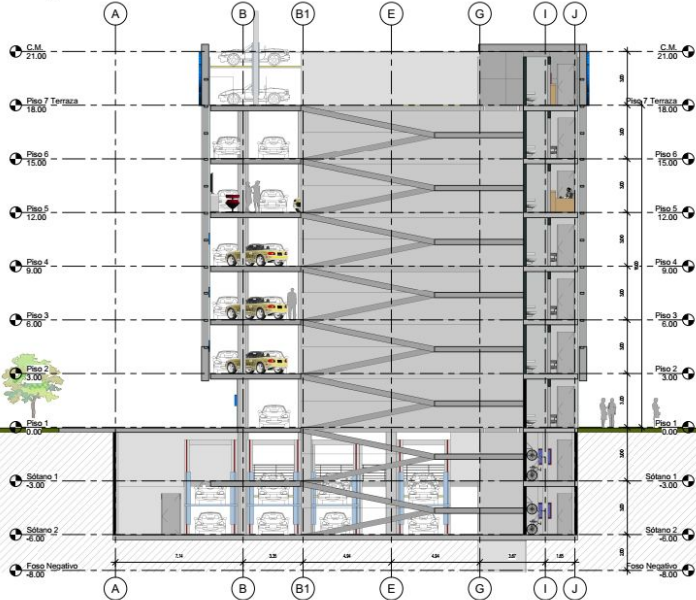
Sección Anométrica Vertical Costado
