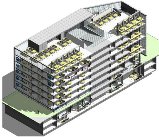
Sección Anométrica Vertical Costado
